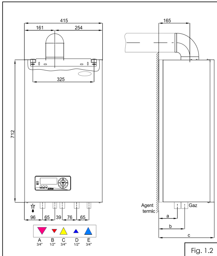
Fig. 1.2 Dimensiuni de gabarit si pozitie de montaj
